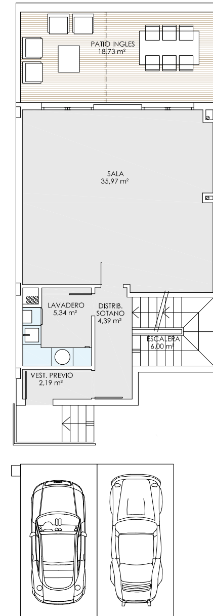
Planta Sótano
