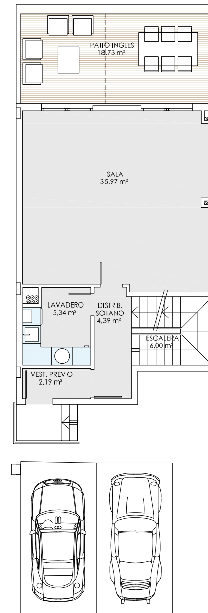
Planta Sótano
